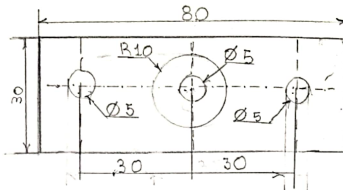
VISTA SUPERIOR
